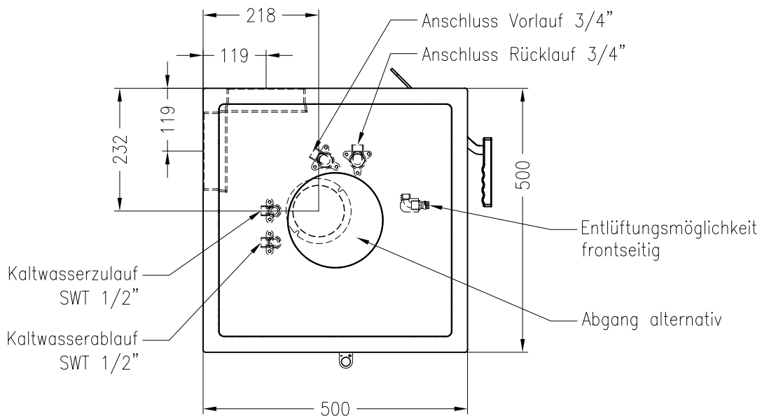
Draufsicht M ~1:10
