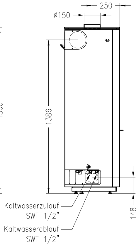
Seitenansicht M ~1:20
